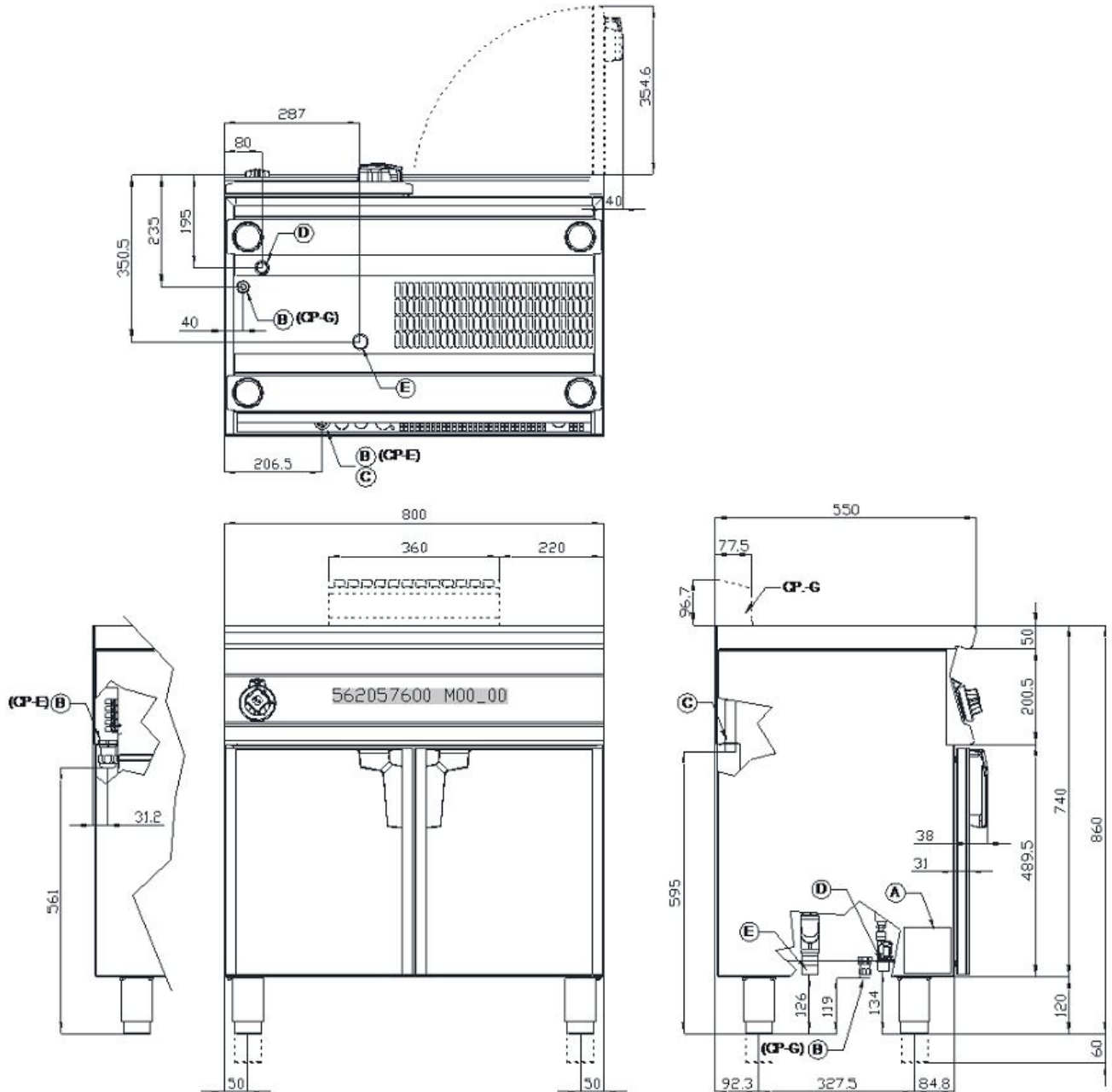
FIG. 1 CP-558G, CPA-558G
