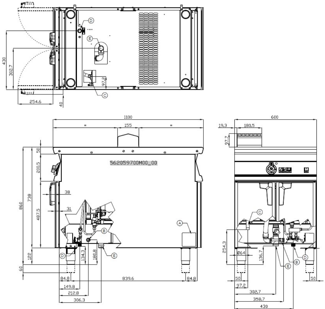
FIG. 2 CP-116G, CPA116G
